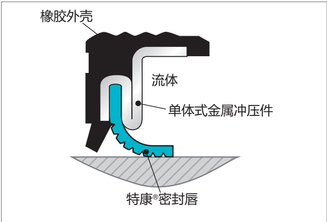
Figure 98: 单壳体设计
