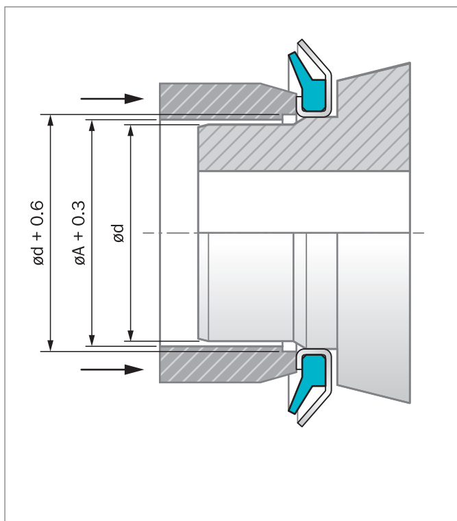
Figure 87: 装配工具。当GAMMA密封件压紧定位台肩时，要注意推力不可太大，以免把壳体压变形。
