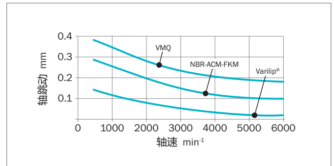
Figure 103: 动态偏心能力
