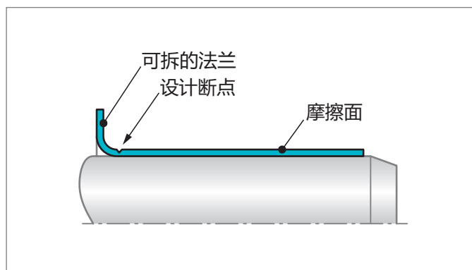
Figure 65: 轴修复套管的设计
