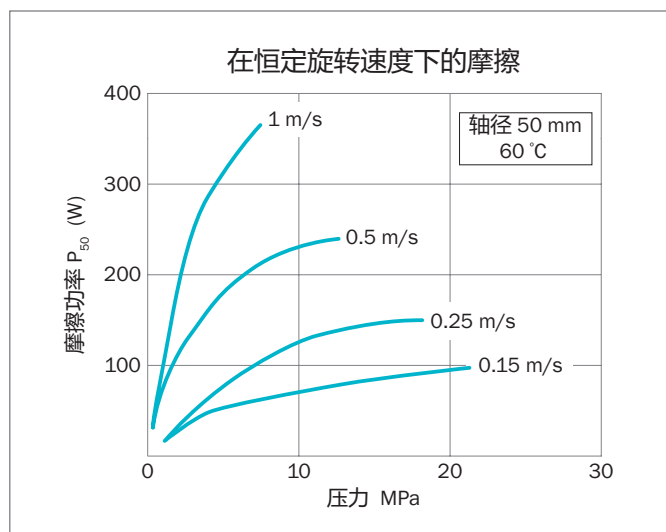
Figure 124: 特康®旋转格来圈®K的摩擦功率
