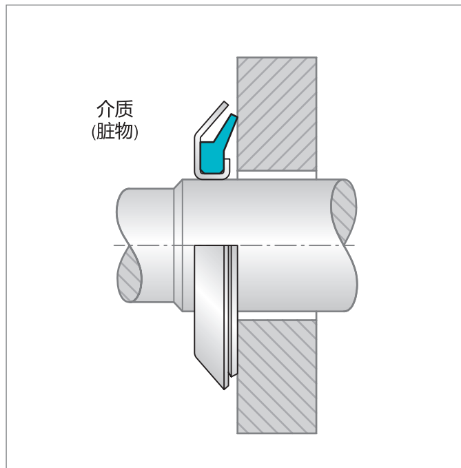
Figure 84: 安装图
