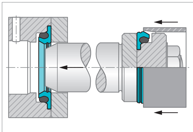
Figure 156: 杆用特康®旋转泛塞®和旋转VL Seal®F在分体式沟槽中的安装
