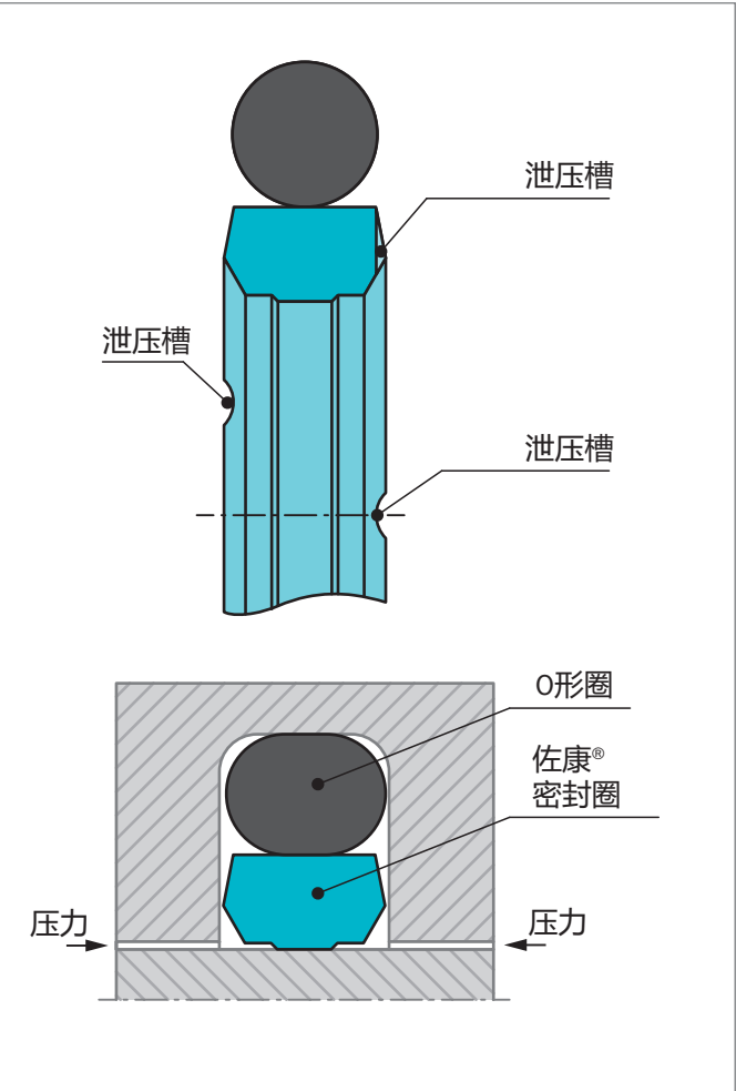
Figure 133 佐康®旋转格来圈®S
