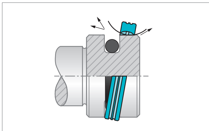
Figure 165: 特康®密封圈的安装示意图
