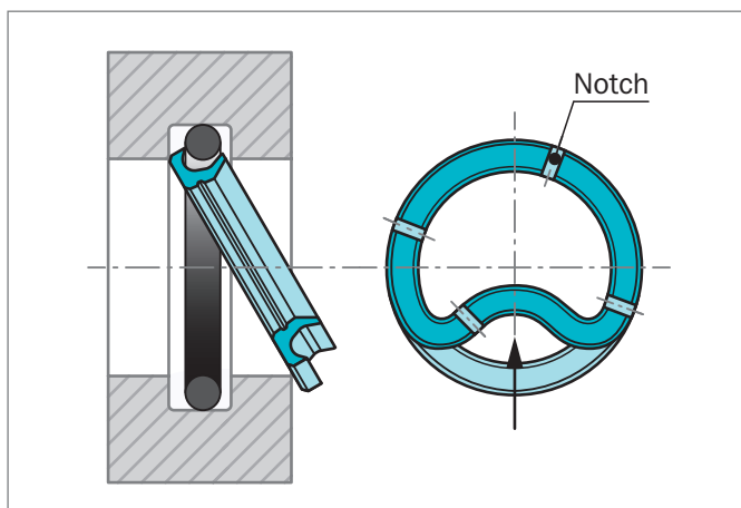
Figure 160: 轴用特康®旋转VL Seal®在密闭式沟槽中的安装
