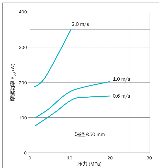
Figure 130 特康®旋转格来圈®V的摩擦功率，特康®M15材料
