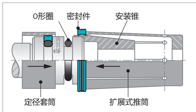
Figure 162: 使用一个扩展式推筒将特康®旋转格来圈®等其它密封件扩展后推过安装锥
