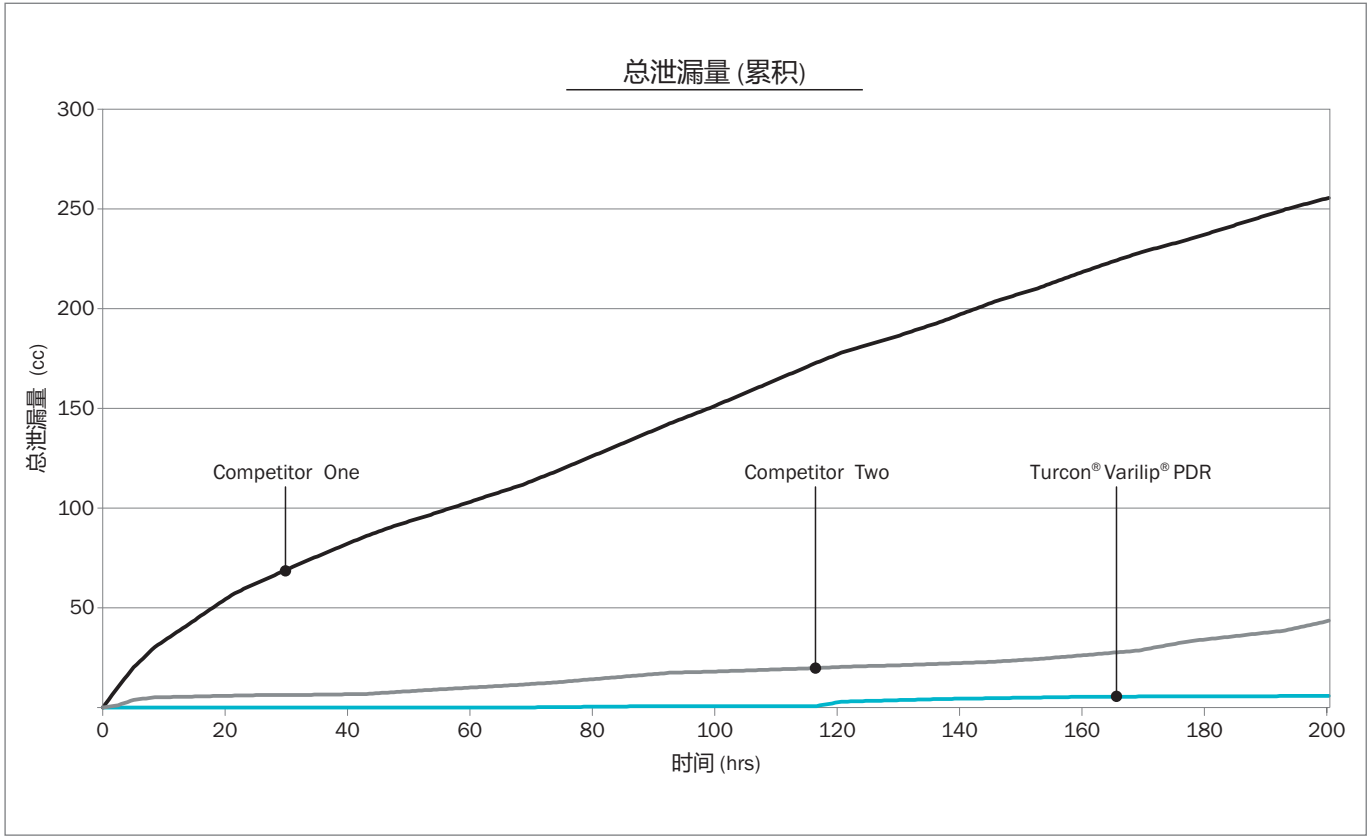
Figure 106: 泄漏总量(累积)，监测200小时以上的试验(平均值)
