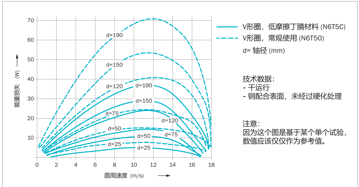
Figure 71: 能量损失和圆周速度的函数关系, 针对各种尺寸
