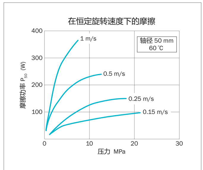
Figure 119: 特康®旋转格来圈®的摩擦功率
