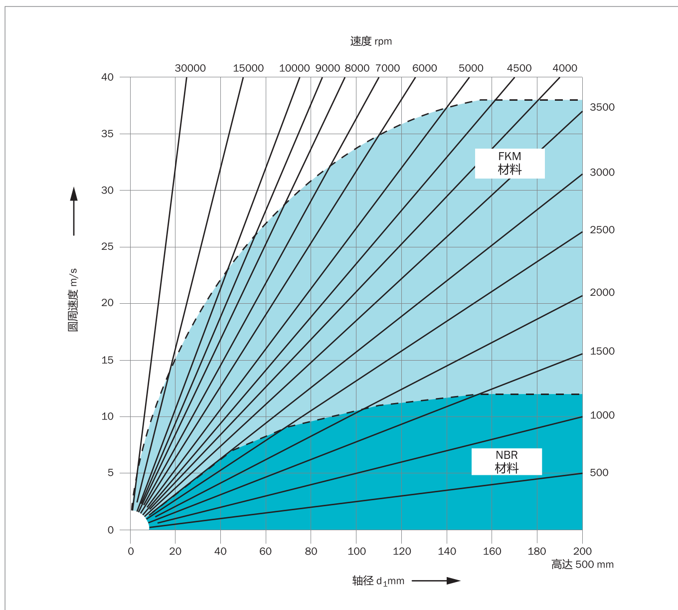
Figure 10: 在无压力状态允许的速度，符合DIN 3761标准
