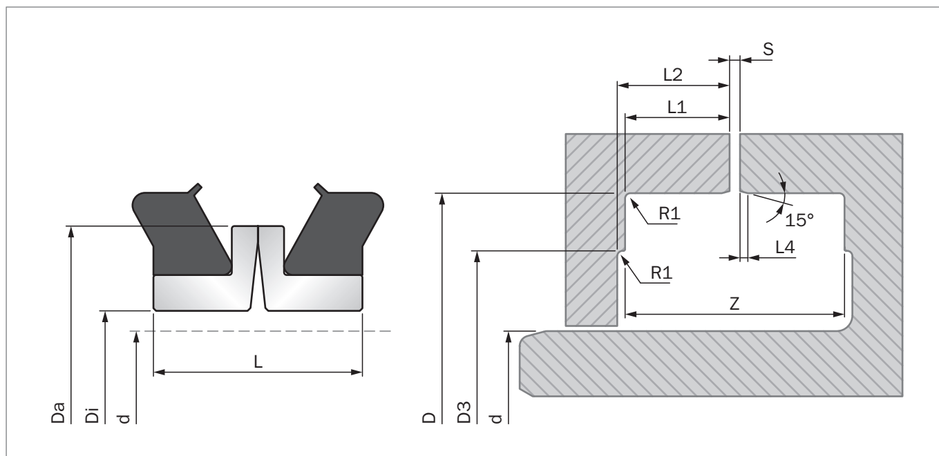
Figure 186: 安装图
