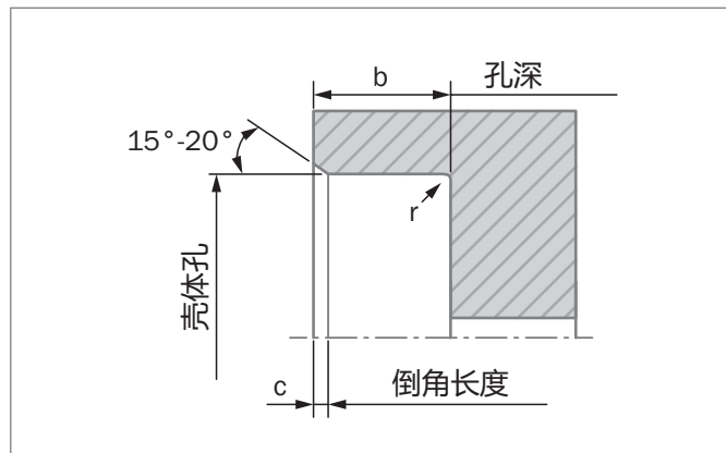
Figure 107: 沟槽设计示意图
