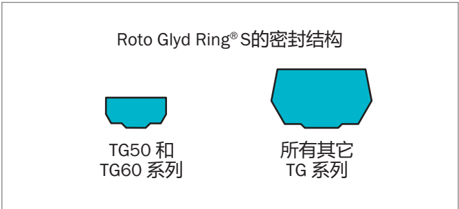
Figure 135 横截面结构根据系列号
