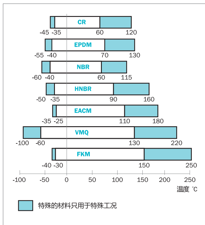
Figure 72: V形圈的温度建议
