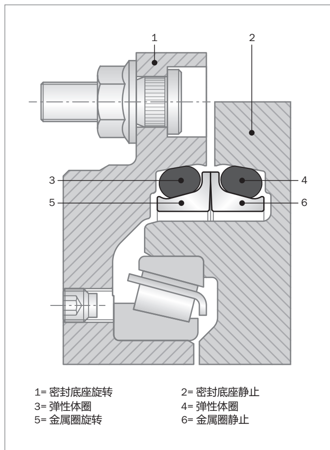
Figure 173: 机械端面密封，DO型
