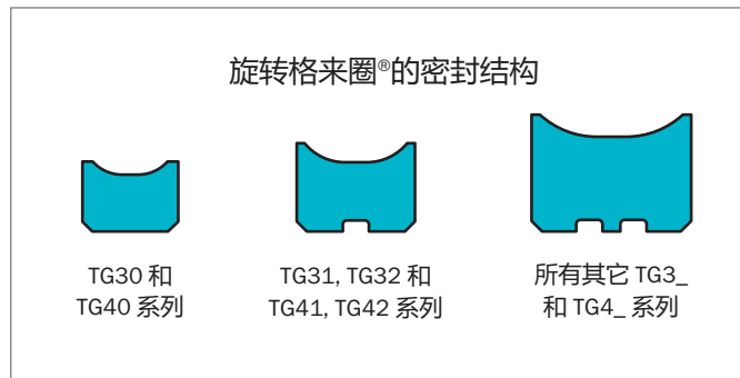
Figure 118: 不同系列号的截面形状
