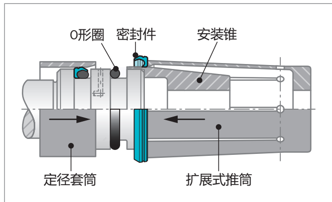
Figure 164: 孔用特康®旋转VL Seal®使用安装锥和扩张推筒进行校准和安装
