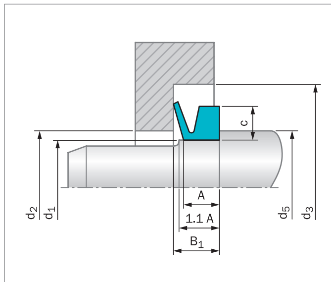
Figure 73: 轴向支承
