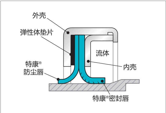
Figure 96: 卡紧式设计
