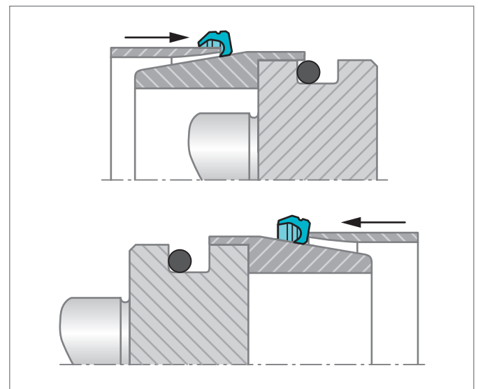
Figure 163: 孔用特康®旋转VL Seal®在密闭式沟槽中的安装, 使用一个扩展式推筒将密封件扩展后推过安装锥。
