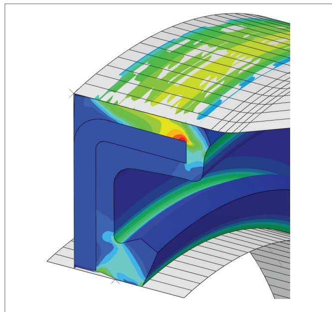
Figure 24: 高压下的有限元分析
