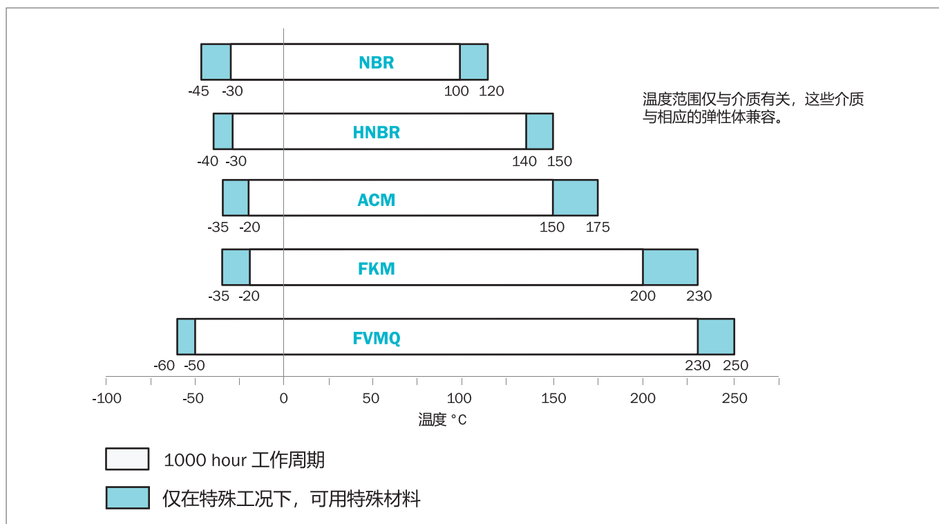
Figure 7: 一些普通橡胶类型的温度限制
