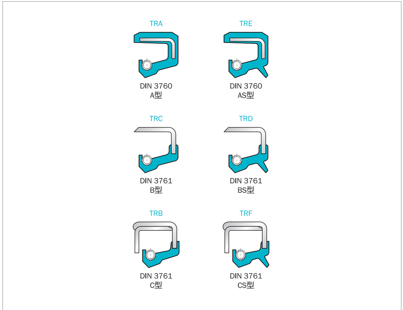
Figure 13: 标准型
