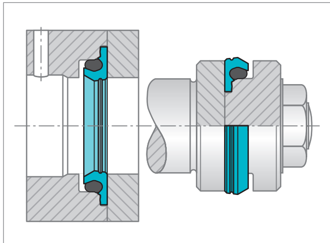
Figure 155: 杆用特康®旋转泛塞®和旋转VL Seal®F在分体式沟槽中的安装
