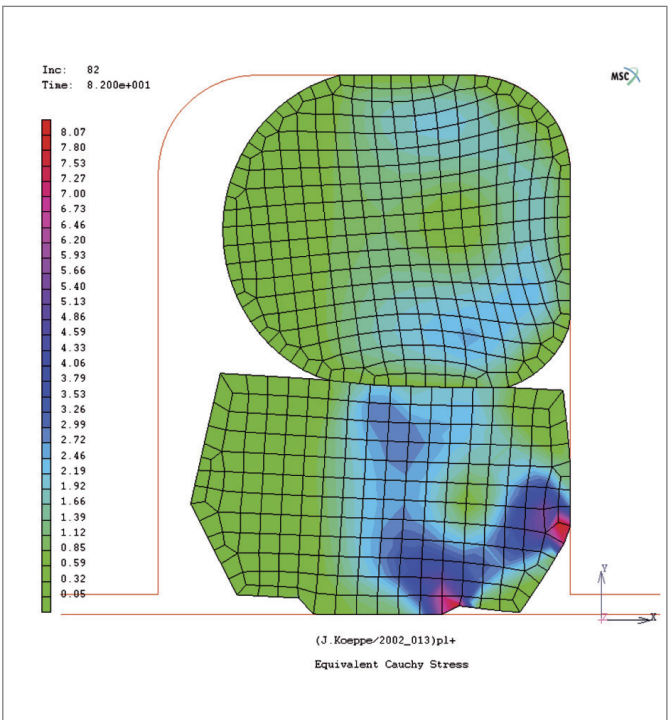
Figure 134 佐康®旋转格来圈®S - 有限元分析
