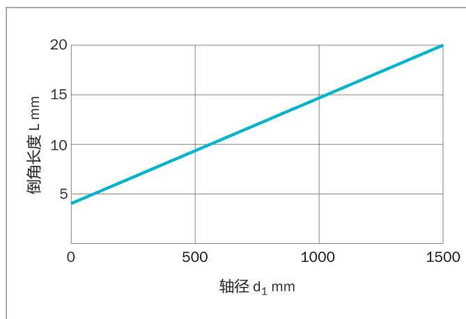
Figure 41: 倒角长度和轴径的函数关系
