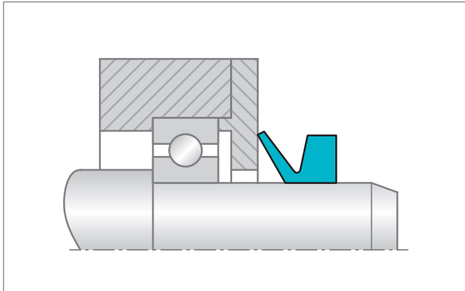
Figure 70: V形圈的工作方式
