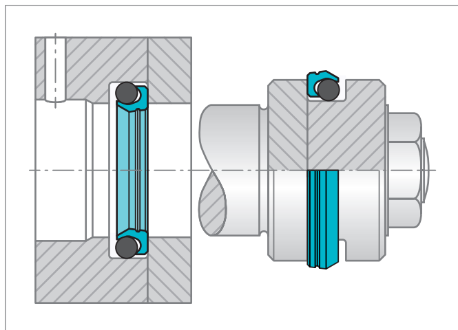
Figure 153: 旋转VL Seal®分体式沟槽中安装
