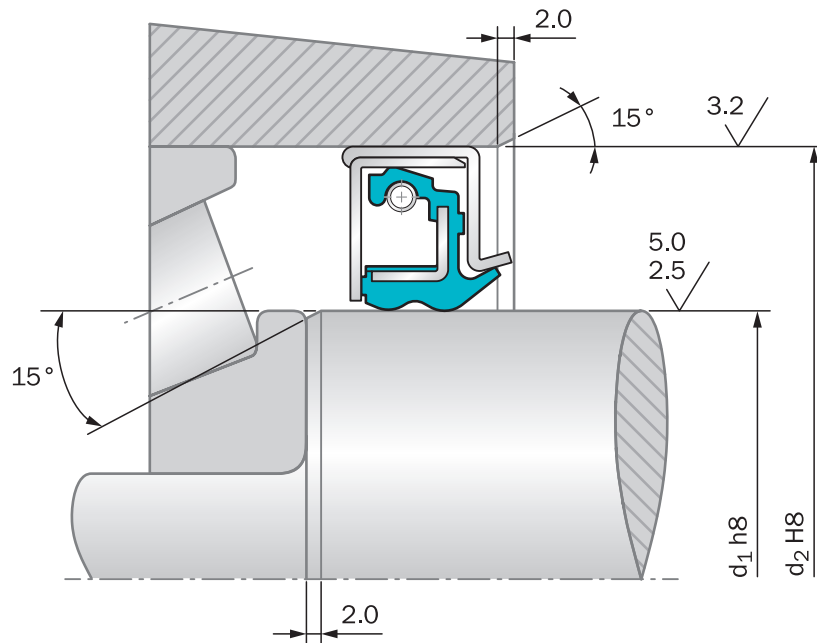
Figure 54: 在轮毂应用中的系统 500 (和系统 2000 和系统 3000相似)
