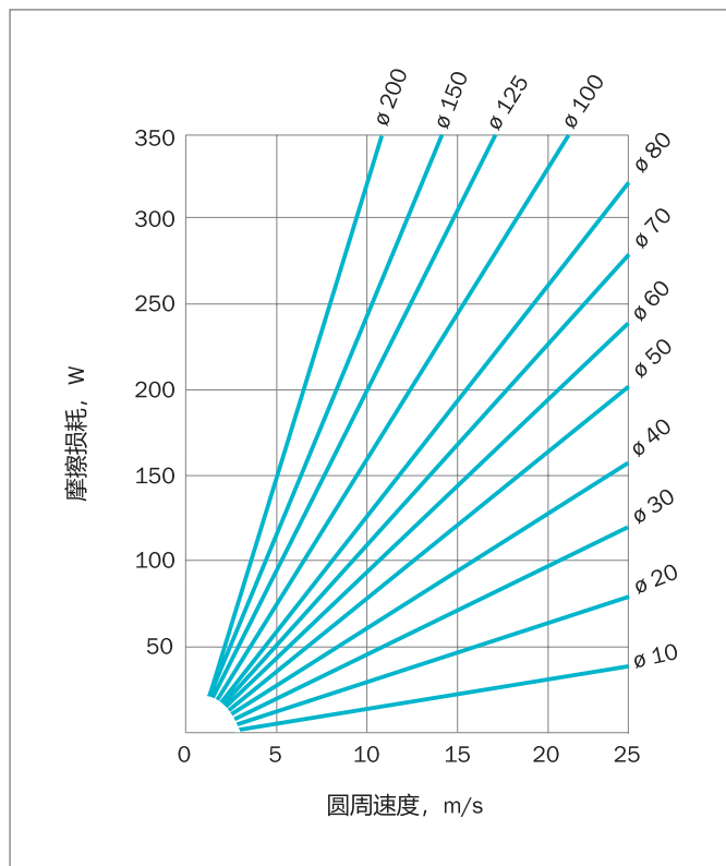
Figure 11: 丁腈材料的TRA型密封件的摩擦损耗
