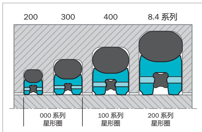
Figure 129 轴用和孔用标准密封系列的截面结构取决于系列号
