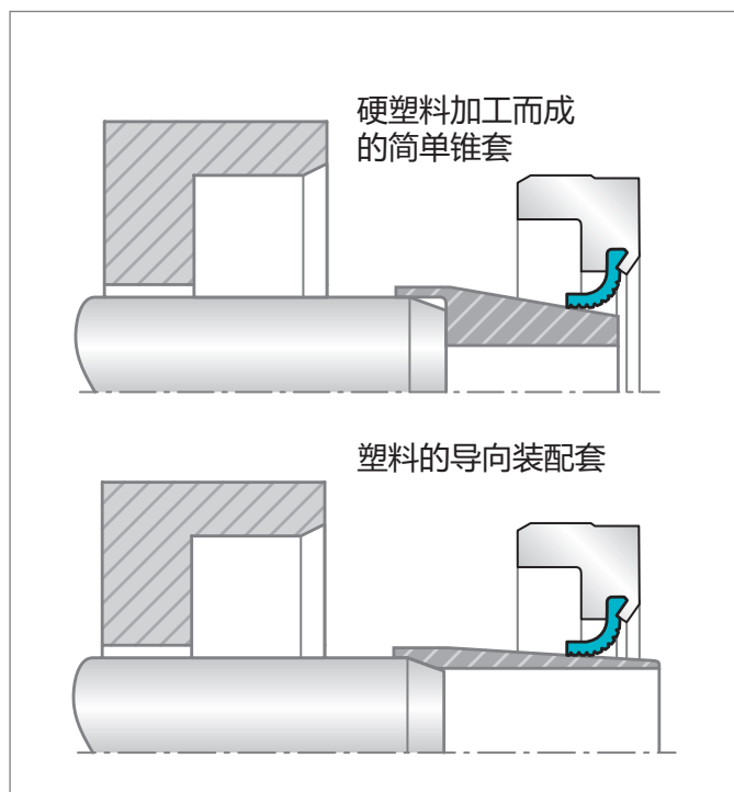
Figure 111: 轴上安装的装配工具类型
