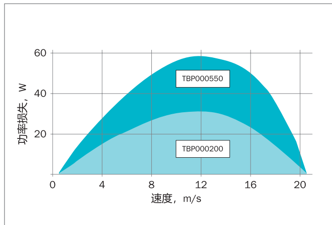
Figure 82: 功率损失和圆周速度的函数关系图 (配合面 1.5 - 2 \mu\text{m} Ra值, 密封件无润滑)
