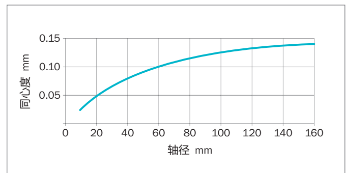
Figure 104: 同轴公差能力
