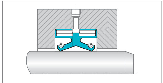
Figure 38: 背靠背装配的TRL型
