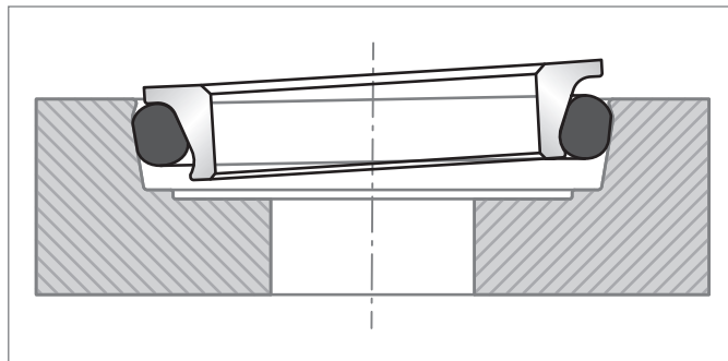
Figure 177: 金属圈向O形圈滑动
