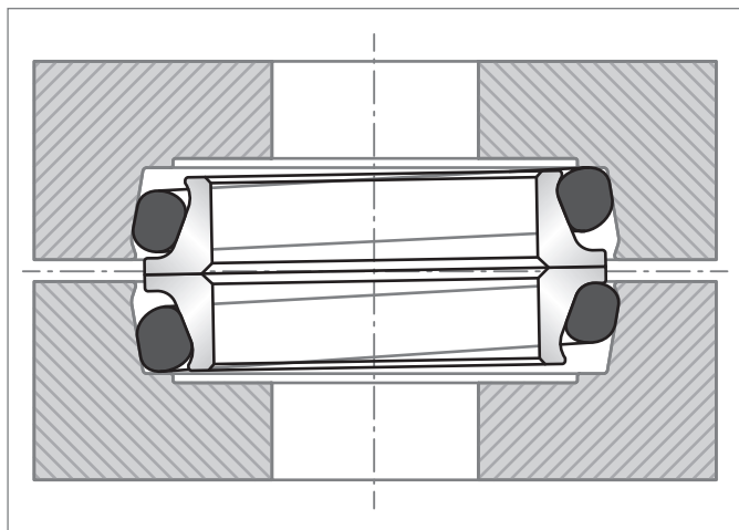
Figure 180: O形圈滑向底座，并且机械端面密封组件倾斜。
