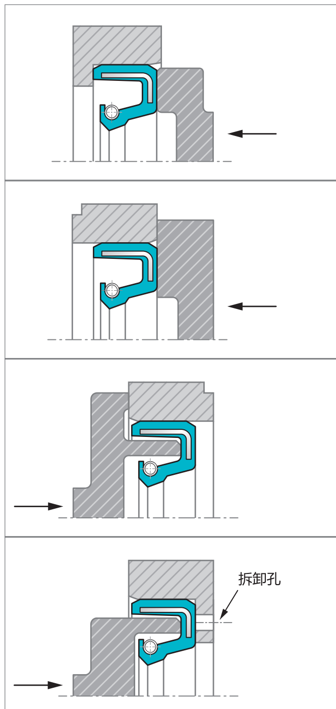
Figure 12: 旋转轴唇形密封件的安装辅助手段
