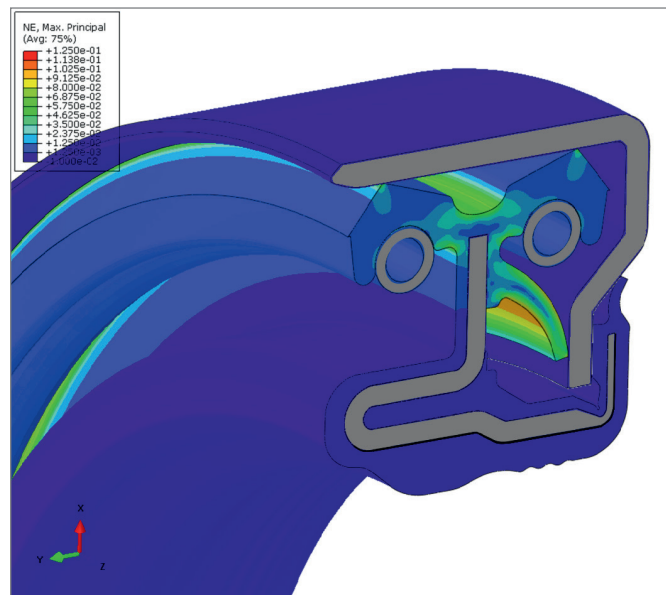
Figure 49: 通过有限元分析FEA，优化摩擦力
