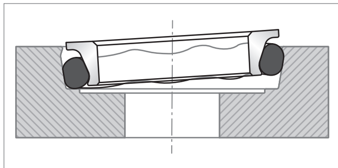
Figure 179: O形圈向底座滑动，并且斜对着金属圈。
