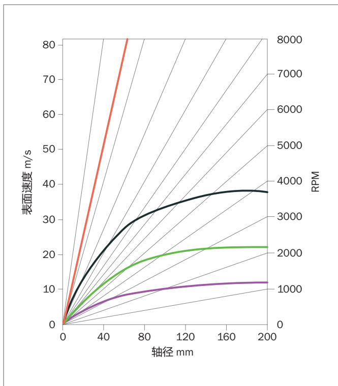
Figure 100: 表面速度和轴径、RPM的函数关系
