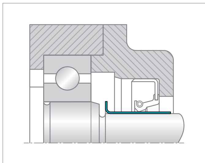
Figure 66: 轴修复套管的摩擦面
