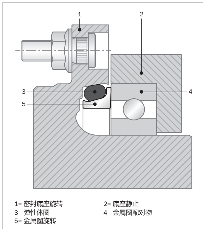
Figure 175: 特殊设计
