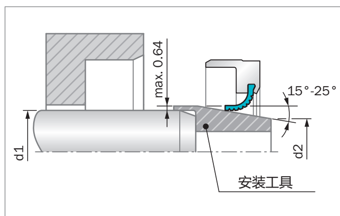
Figure 110: 使用安装工具装配密封唇
