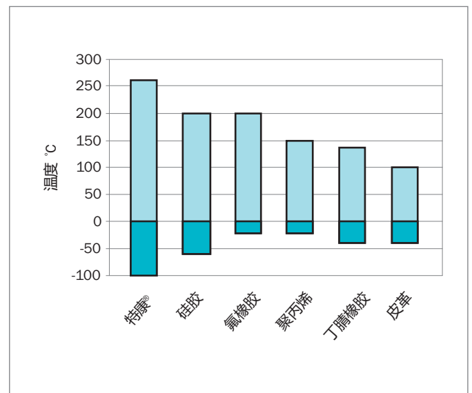
Figure 101: 不同材料的最高和最低温度
