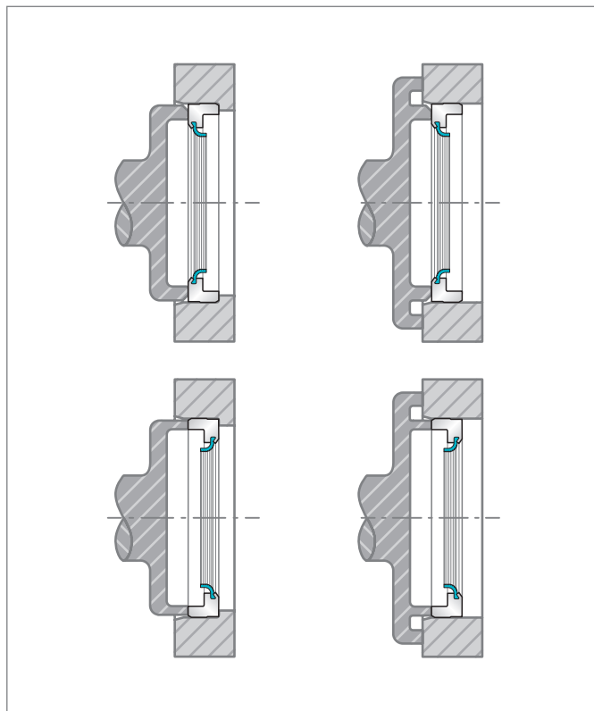
Figure 112: 压入沟槽中的装配工具类型
