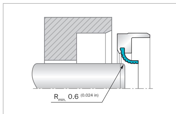
Figure 108: 对于有压力的应用，密封唇背朝轴来安装
