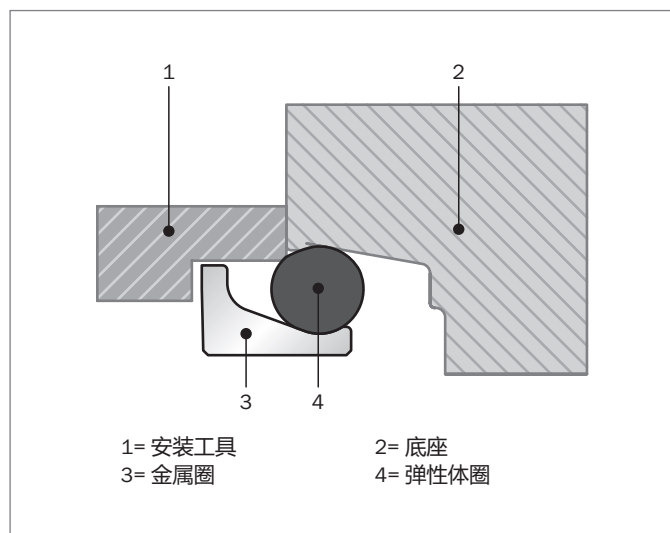
Figure 176: D0型安装工具
