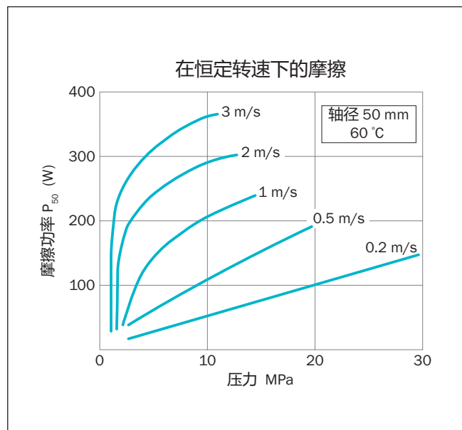
Figure 144: 特康®旋转VL Seal®F的摩擦功率
