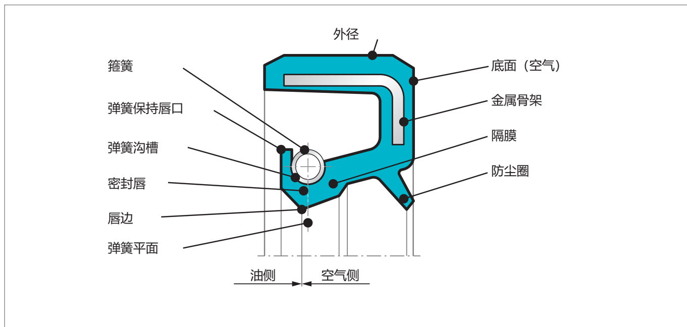
Figure 1: 旋转轴唇形密封件的名称构造 (源自ISO 6194)
