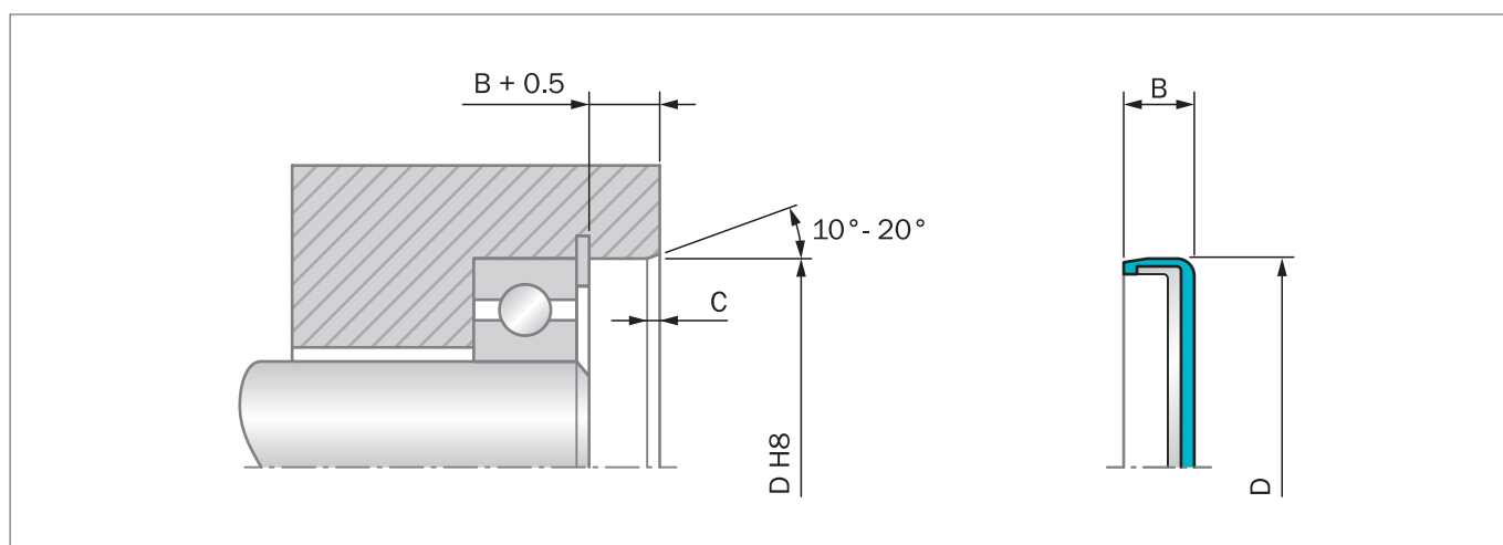
Figure 63: 安装图
