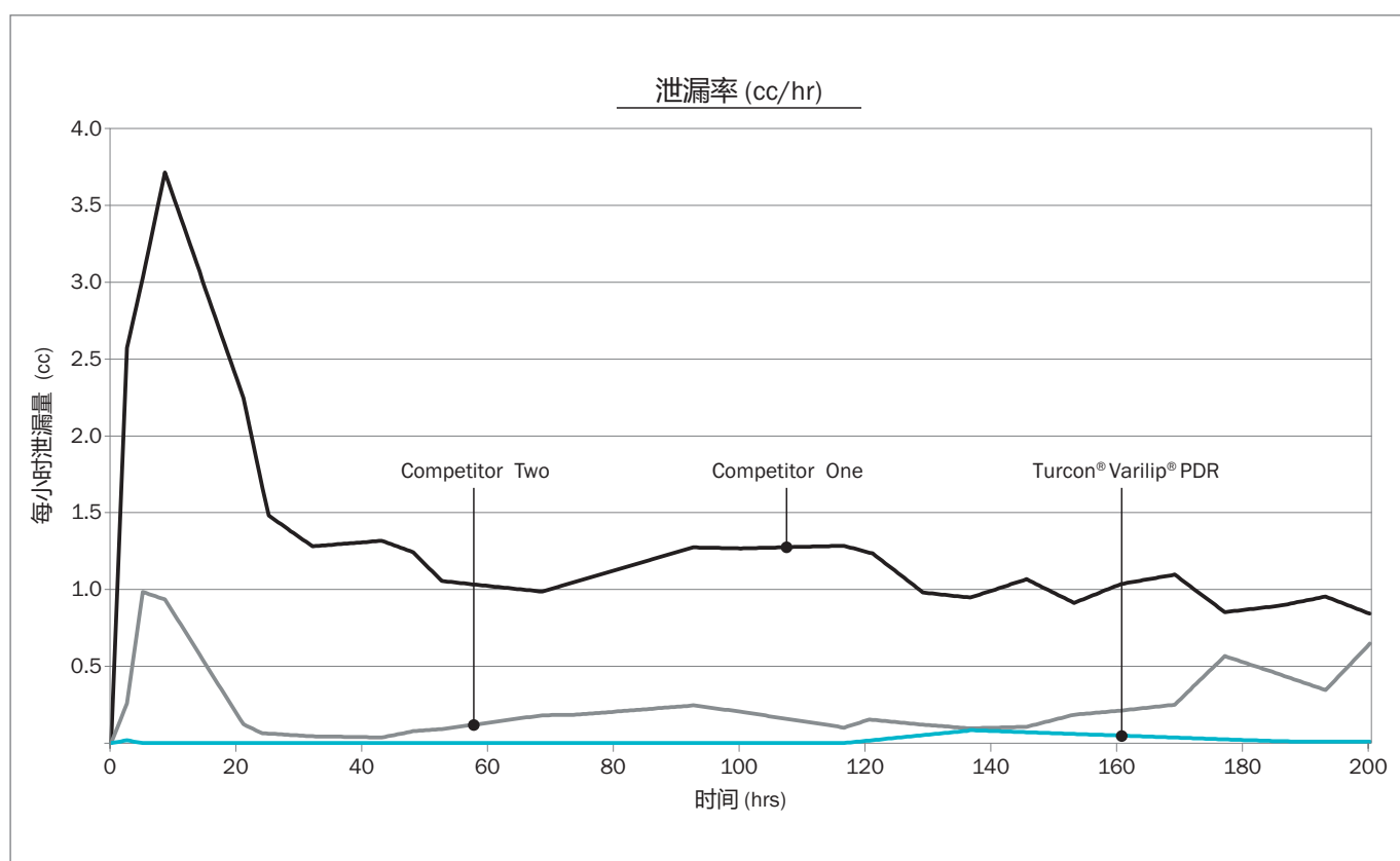
Figure 105: 每小时的泄漏量，监测200小时以上的试验(平均值)
