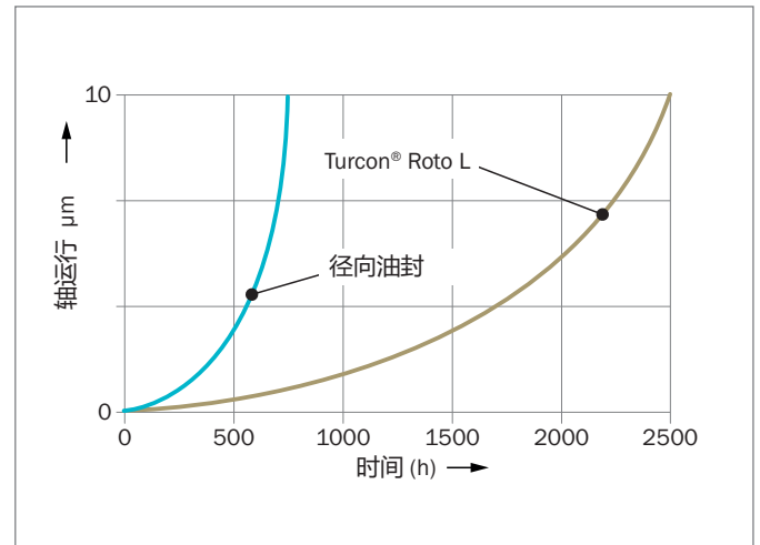
Figure 94: 硬件使用寿命
