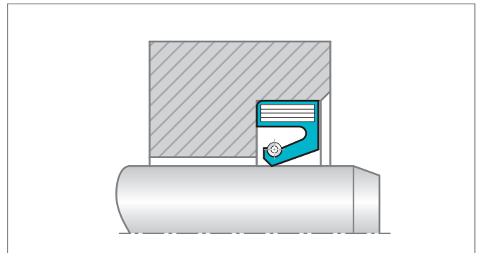
Figure 39: 不带轴向固定板装配的TRJ/F型
