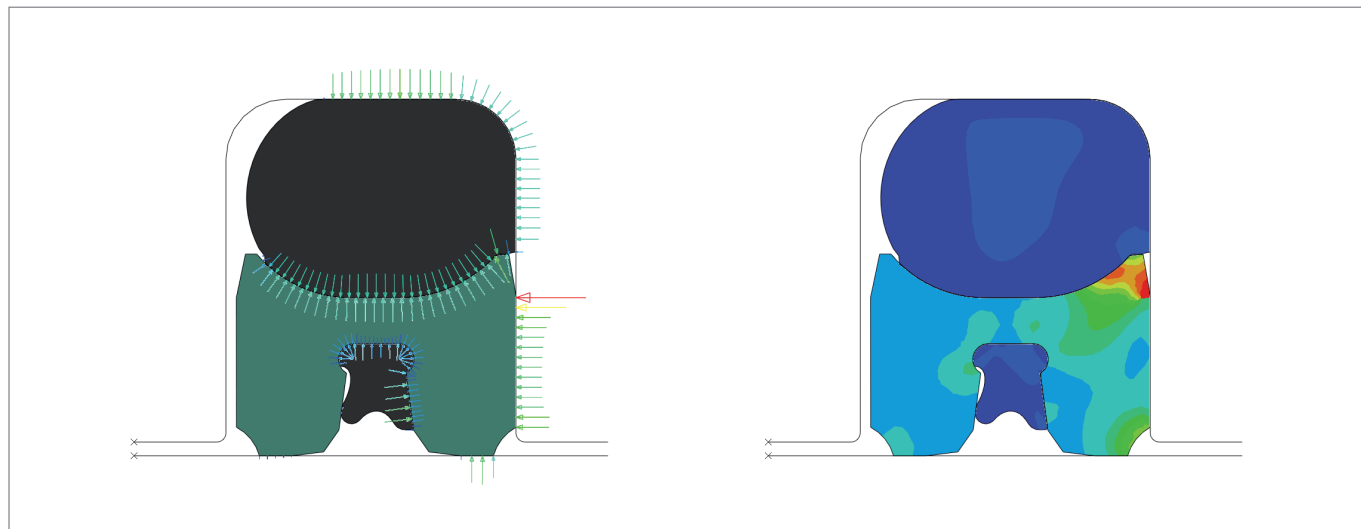
Figure 128 特康®旋转格来圈®V - 有限元分析 (FEA)
