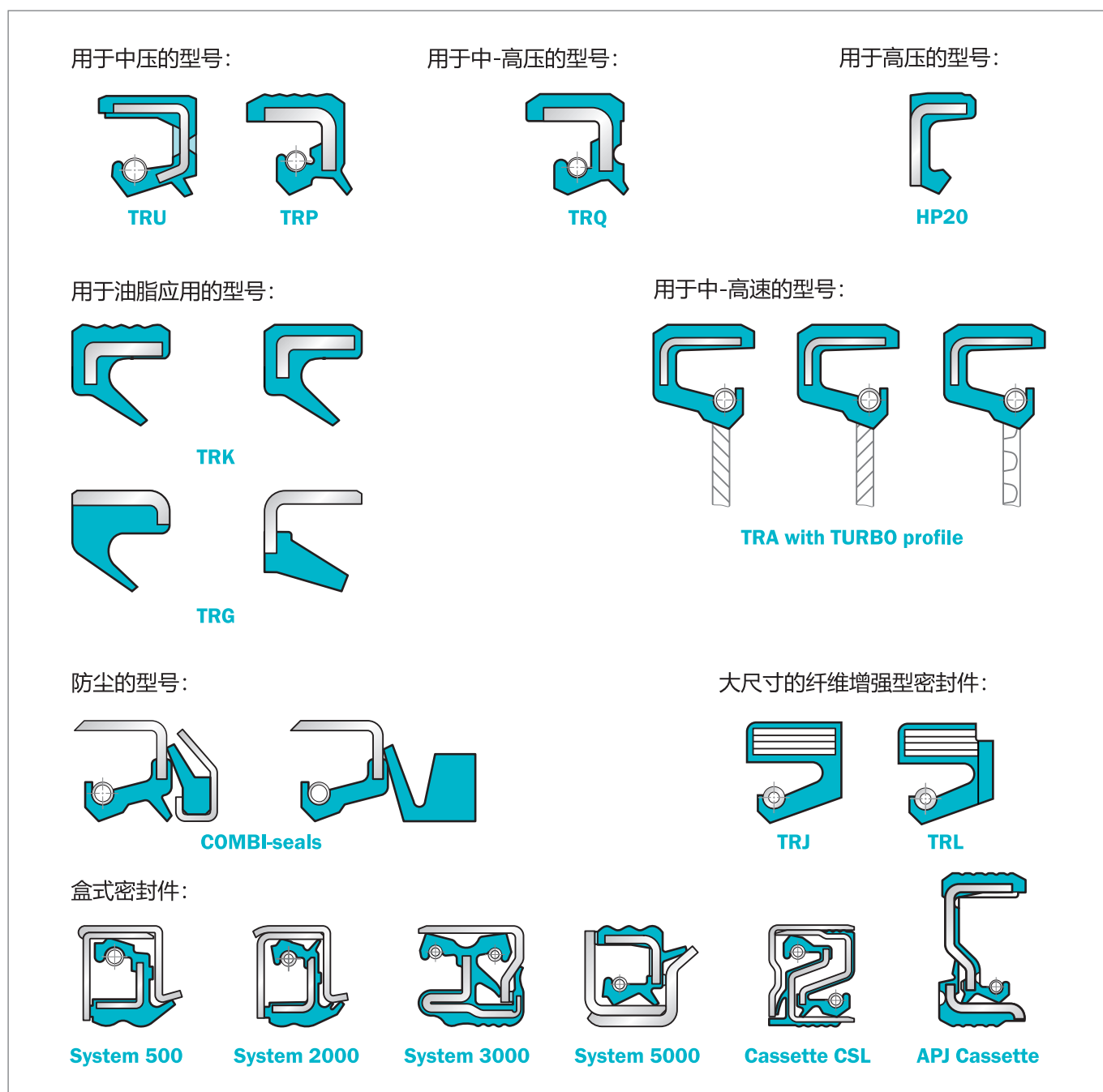
Figure 20: 特殊径向密封件的选择
