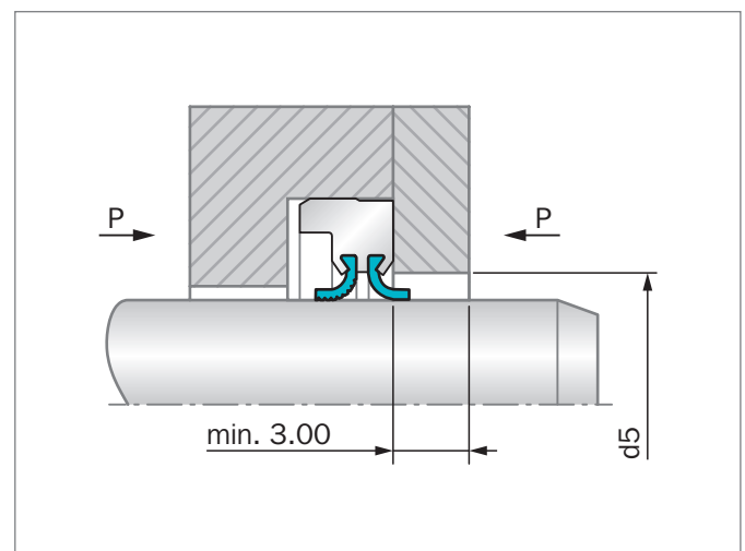
Figure 115: 压力高力0.5 MPa (145 psi), 针对流体分离的安装类型
