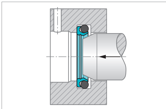
Figure 161: 旋转VL Seal®安装后的校准方向
