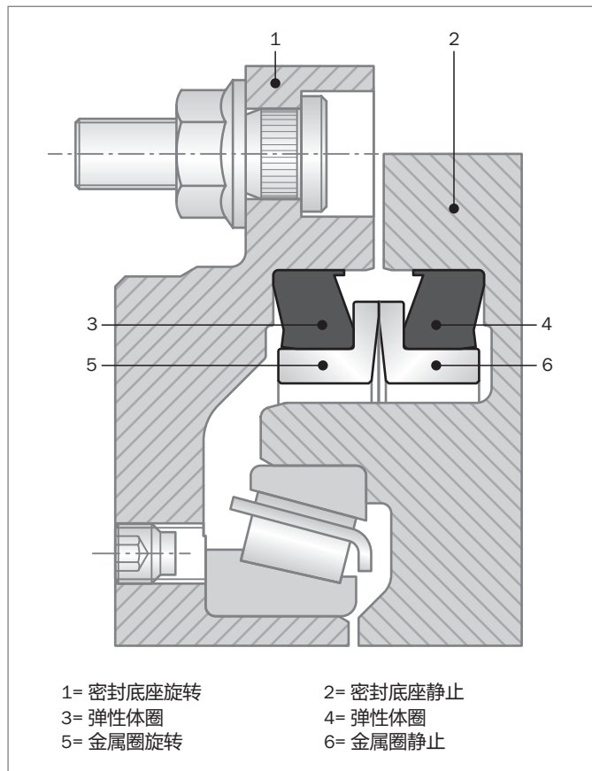
Figure 174: 机械端面密封，DF型
