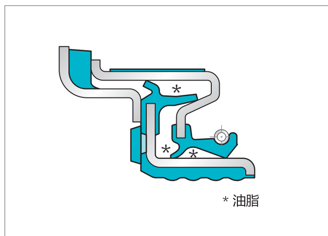
Figure 62: API用于严重污染的应用和轴向作用
