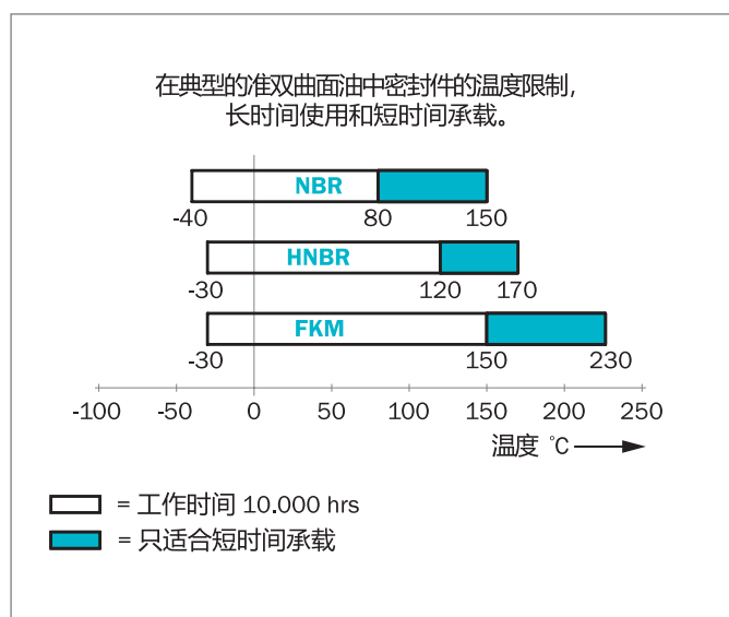
Figure 53: 温度建议，在典型准双曲面齿轮油中
