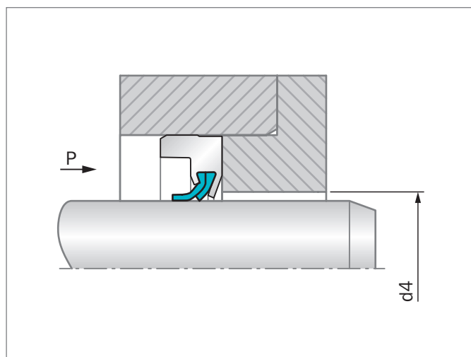
Figure 114: 压力范围在0.5 MPa (73 psi) ~ 1 MPa (145 psi) 的安装图纸
