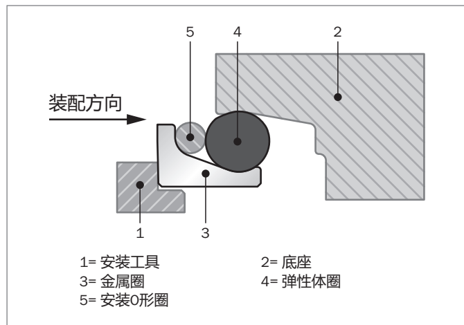
Figure 183: O形圈作为安装工具
