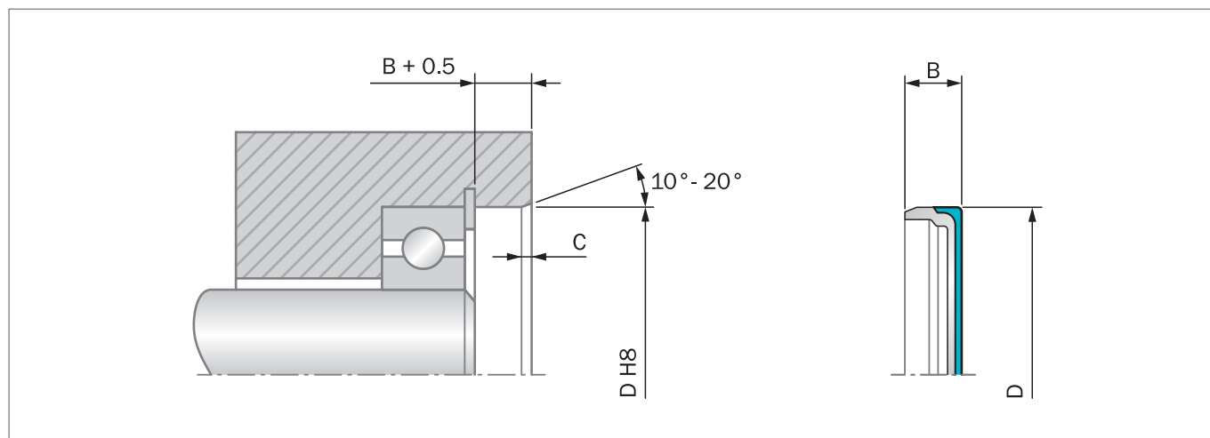
Figure 64: 安装图
