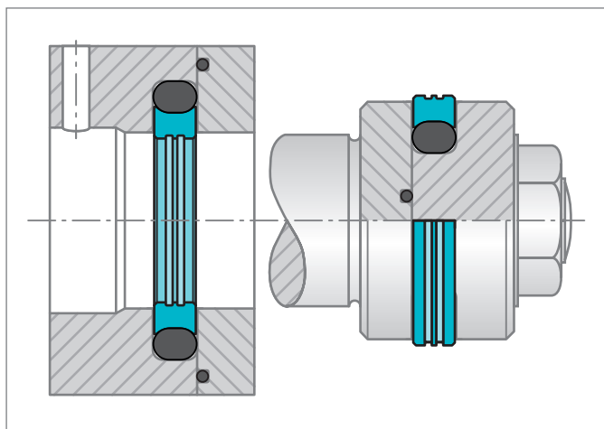
Figure 152: 旋转格来圈®分体式沟槽中安装
