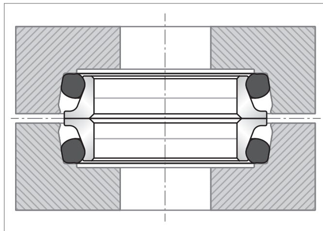
Figure 182: 机械端面密封组件的上下对等部分的O形圈均滑向底座，并且位于底座底部。
