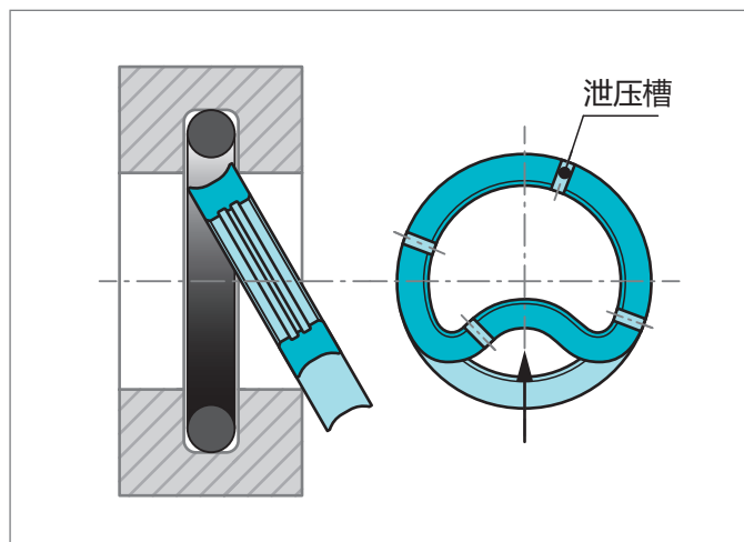
Figure 157: 轴用旋转格来圈®在密闭式沟槽中的安装
