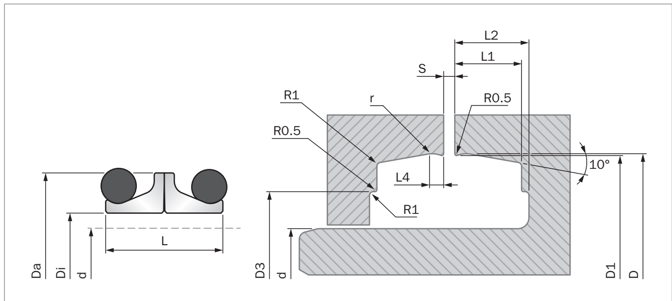
Figure 185: 安装图
