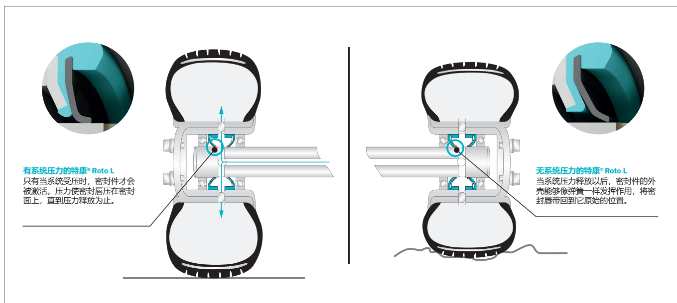
Figure 92: 特康®Roto L的工作原理
